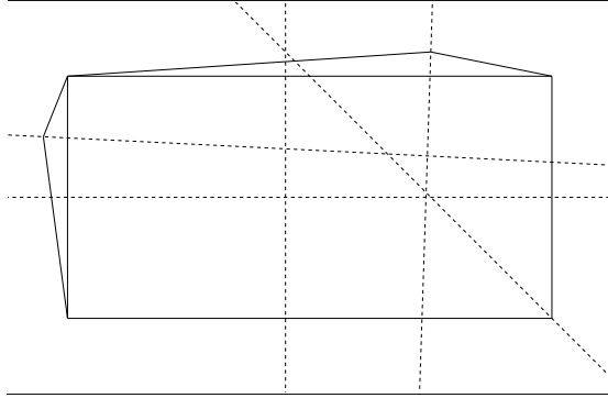
Fig. 2 The heart of Q_\varepsilon .
